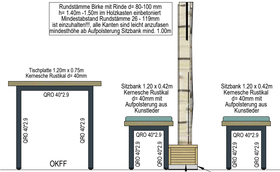
Ansicht
