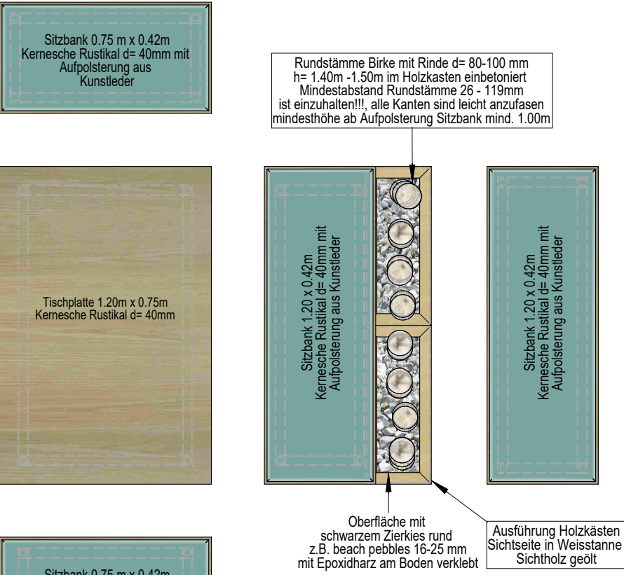
Grundriss
